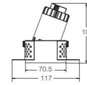
Ø 117mm ( \varnothing 82)
