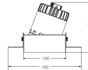
Ø 162mm ( \varnothing 102*102)
