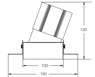
Ø 162mm ( \varnothing 102*102)
